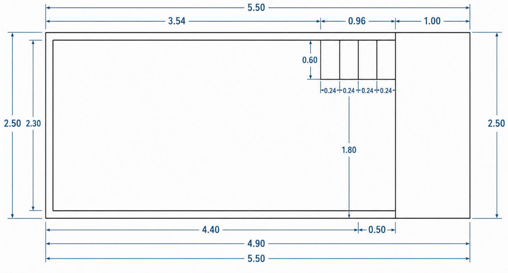
PLANTA SUPERIOR
